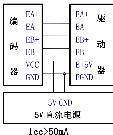
编码器外加电源供电时接线图
